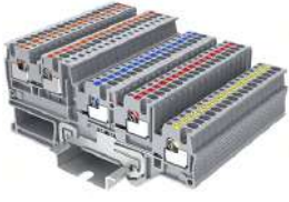
TPIO1.5-S-4-PE
