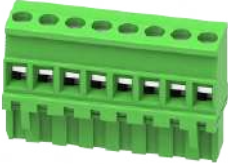
MC-RE5.08V08C-0001
