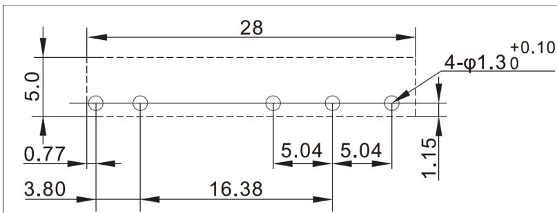
PCB kart dizaynı için çizim
