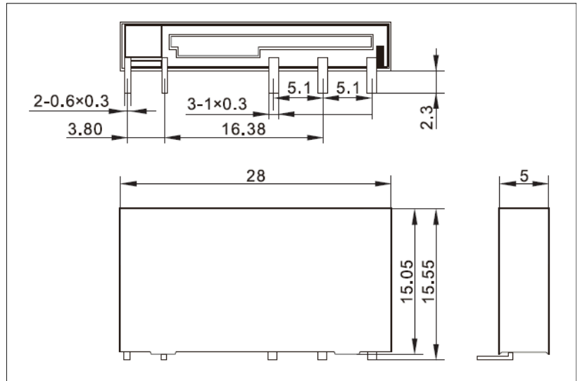
Yatay düzlem çizimi (Pimlerle birlikte)
