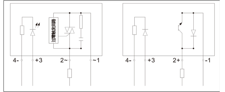
Kablolama Şeması
