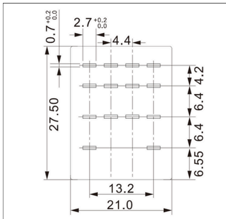
PCB kart dizaynı için çizim
