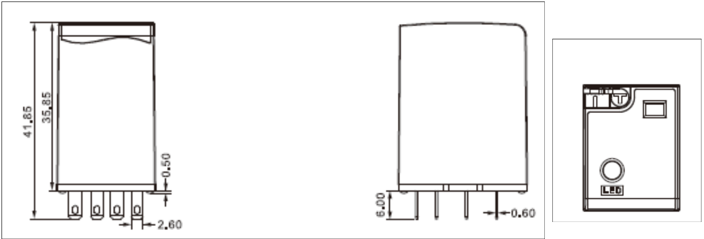
Dikey düzlem çizimi (Pimlerle birlikte)
