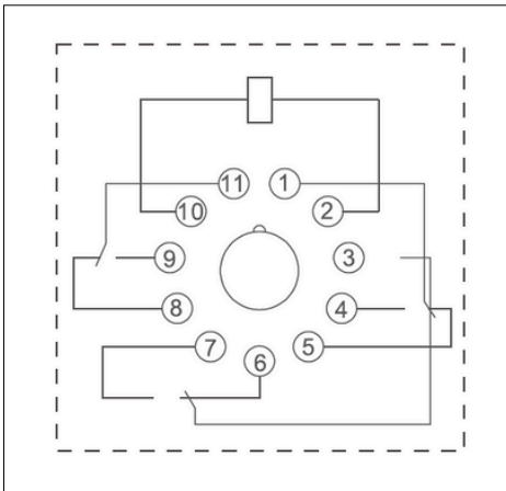
Kablolama Şeması
