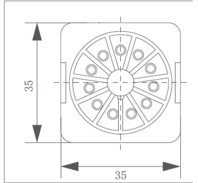
Pinlerin Çizimi
